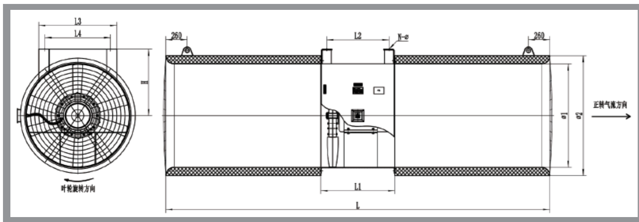
射流风机外形尺寸
